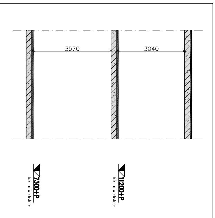
Doorsnede
